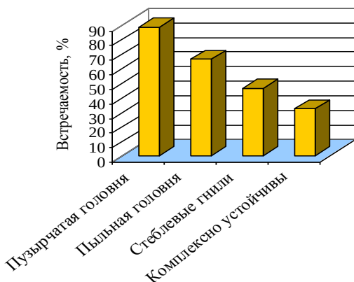
Рисунок 8. Комплексная иммунологическая оценка линий, описанных в литературе в качестве источников устойчивости к пузырчатой головне.
