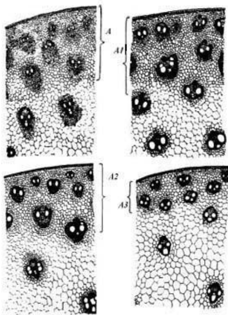
Рисунок 11. Анатомические особенности строения коры стеблей (x 50): А – толщина коры и характер её склерификации у теосинте; А1 – у гибрида Од301 x В1Р133; А2 – у самоопыленной линии В1Р 44; А3 – у линии Д-6-2-5-5-1-2 (ориг.)
